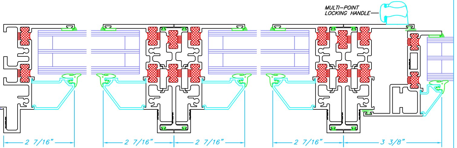
8 JAMB Ⓞ FIXED
